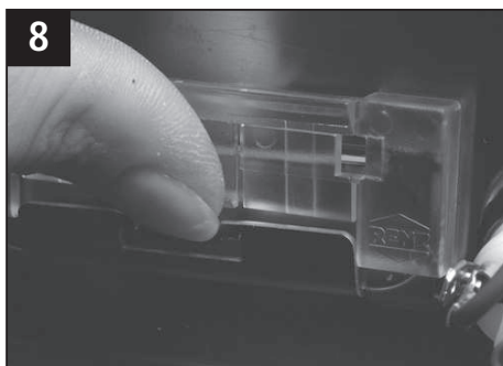
8 Halter mittig nach hinten drücken und gleichzeitig nach oben herausziehen.
