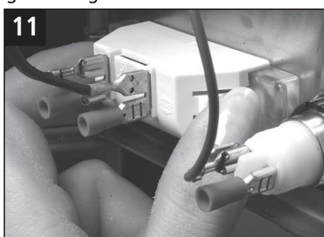
11 Beleuchtungshalter aufstecken.
